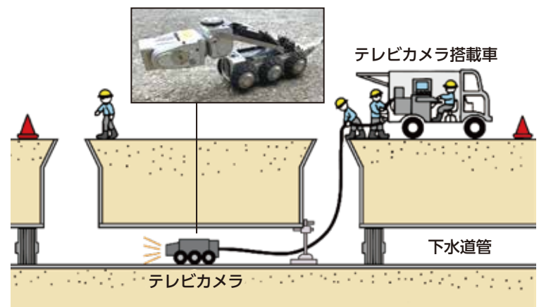
▲老朽管のカメラ調査
