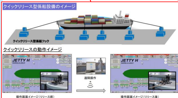
図 クイックリリース型係留設備
