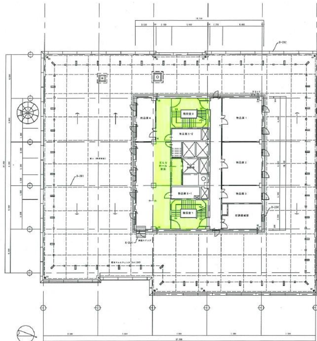
5階 平面図 ①～⑤：物産室の配置図 ⑥～⑧：上記以外の配置図
