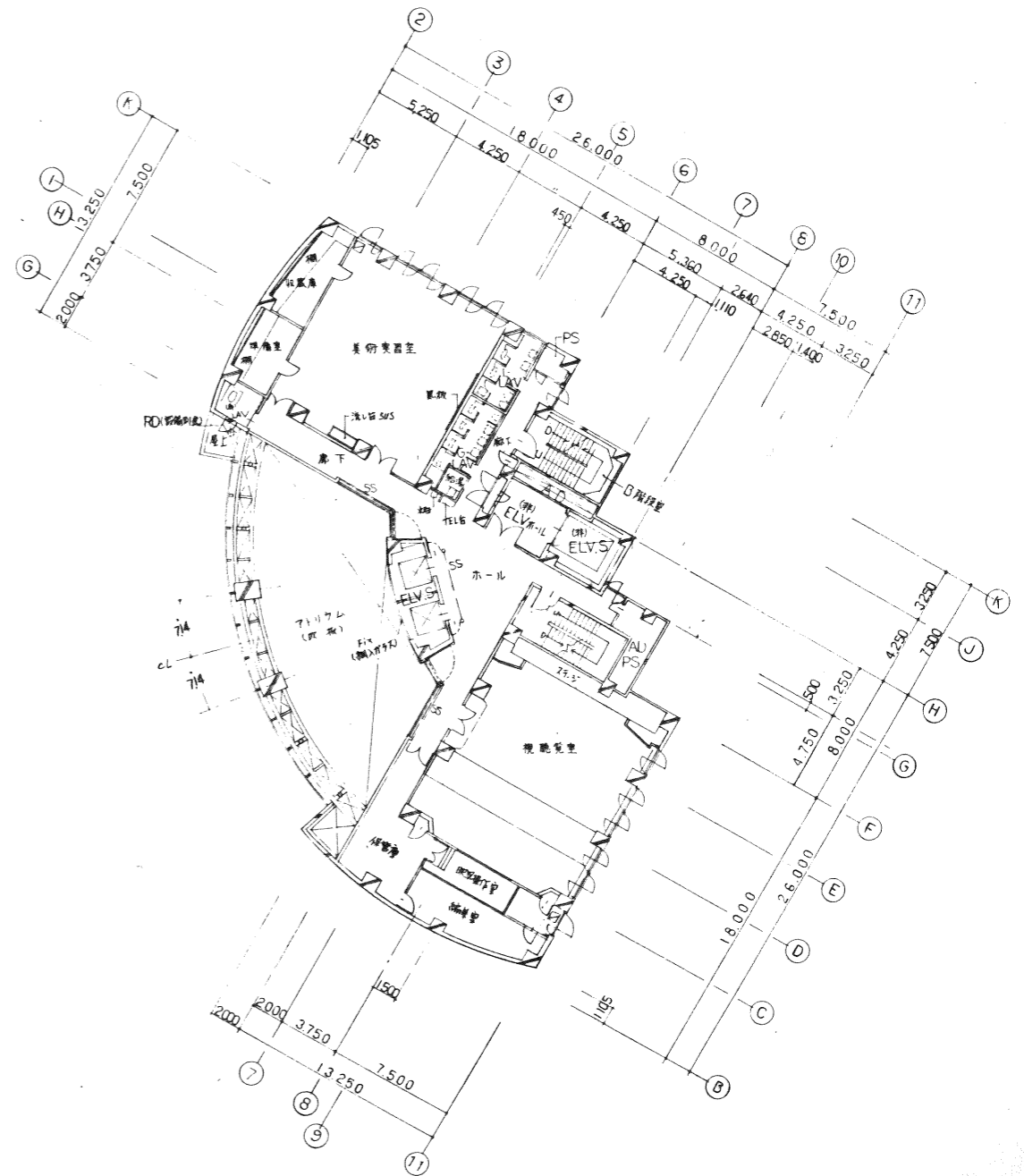
5階平面図 S=1:200
