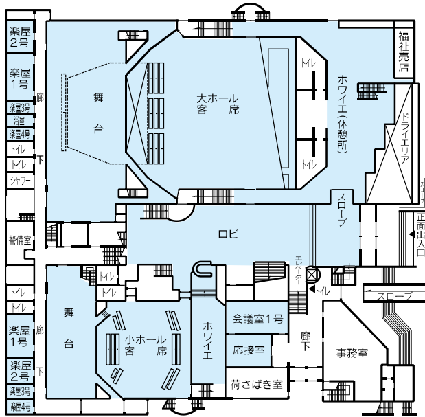
1階平面図
