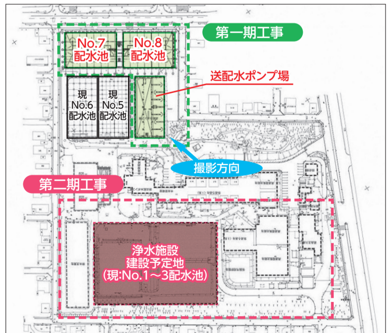
▲愛国浄水場内見取図
