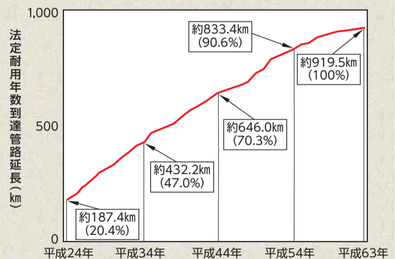
釧路市の水道管路が法定耐用年数(40年)に到達する時期 ※平成23年度末釧路地区現存水道管路の更新を行わない場合。
