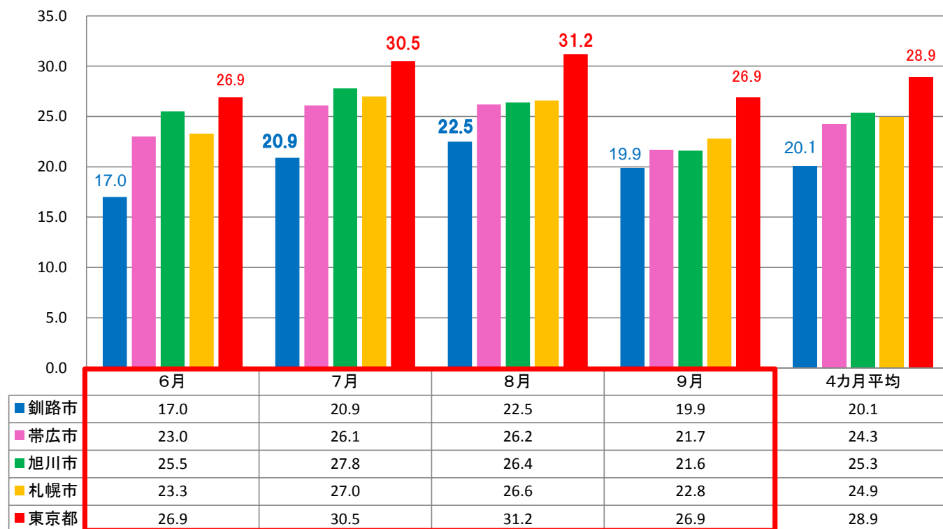
平成26年度の日最高気温の月平均値(℃) (気象庁ホームページより)
